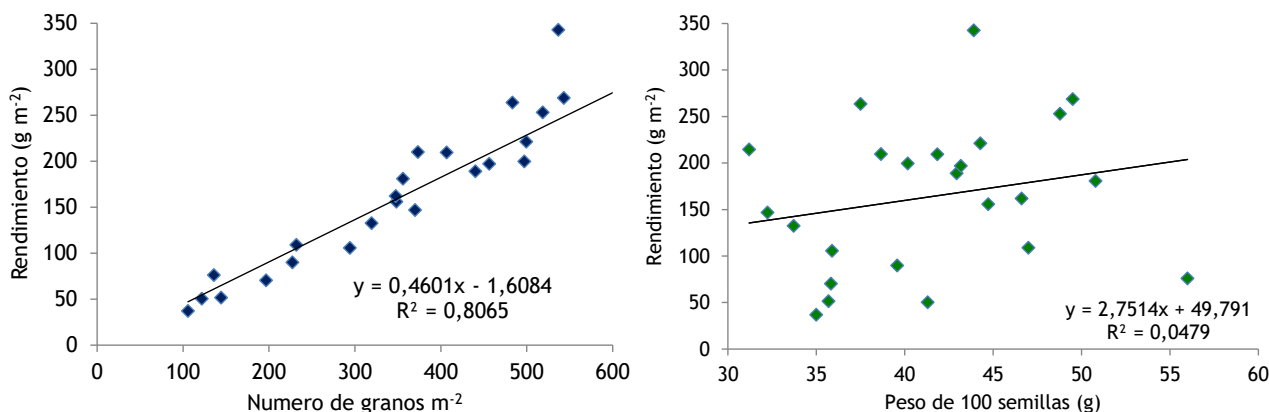
Figura 6: Relación del rendimiento (expresado en \text{g m}^{-2} ) de la variedad Norteño a) con el número de granos y b) con el peso de 100 granos, campañas 2011/12 al 2017/18. Campo Escuela, FCA-UNC. ( 31^{\circ}19'LS , 64^{\circ}13'LV ) (Toledo, 2018)
