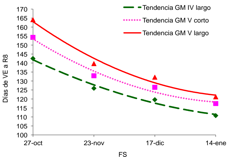
Figura 7: Tendencia del efecto de la FS sobre el ciclo según GM.
